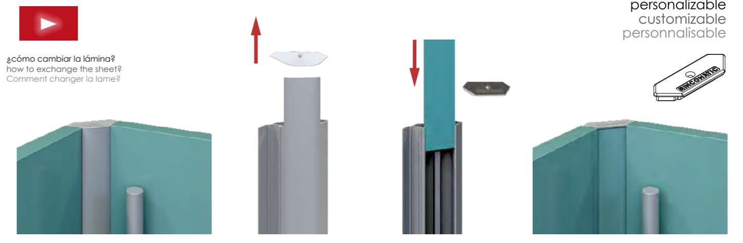
Rincobasic40 incluye terminales rectos y un sistema ajustable que permiten su personalización insertando una lámina decorativa plana (ancho 31mm; grosor de 0,4 a 2 mm) Rincobasic40 includes straight caps and an adjustable system which allows to customize it by inserting a decorative flat sheet, (width 31 mm; thickness from 0,4 to 2 mm) Rincobasic40 inclut des embouts carrés, et un système adaptable, permettant sa personnalisation grâce à une plaque laminée decorative plate (largeur 31 mm, épaisseur de 0,4 à 2 mm)
